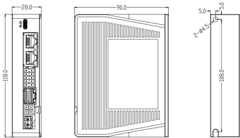
图 2-1 CL3B-EC503/507 安装尺寸图(单位: mm) ※ 设计安装尺寸时, 注意考虑端子大小及布线!
