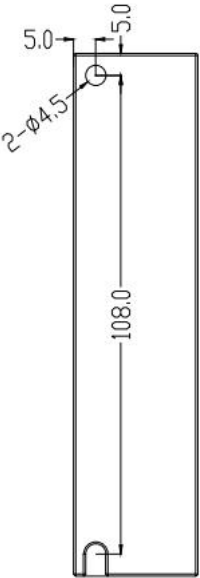
图 2-1 CL3B-EC503/CL3B-EC507 安装尺寸图(单位：mm) ※ 设计安装尺寸时，注意考虑端子大小及布线！
